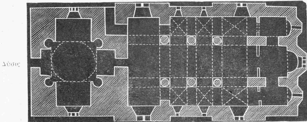
Κάτωψις τοῦ ἐν Πόρτα-Παναγιᾶ Ναοῦ. Κλίμαξ 1/200
