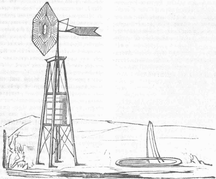
Ἀνεμοκίνητος ὕδραντλία.
