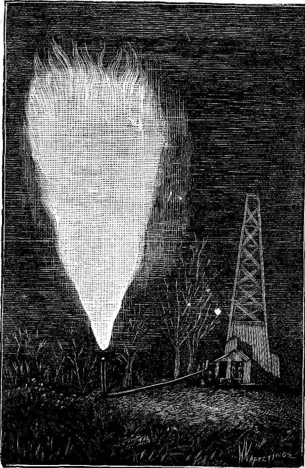
Φυσικὴ πηγὴ φωταερίου καὶ ἰόντος.
